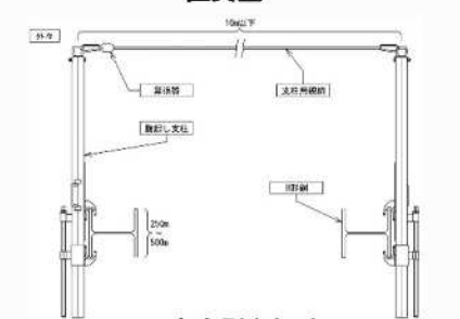
直交型(外々)
