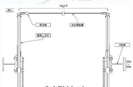
直交型(内々)
